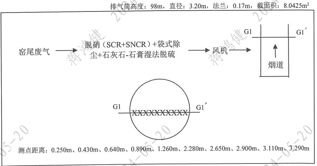
图 1 有组织废气 G1 监测点示意图
